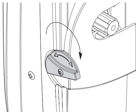
Déblocage pour manœuvre manuelle
