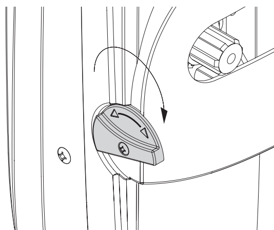
Desbloqueo para maniobra manual
